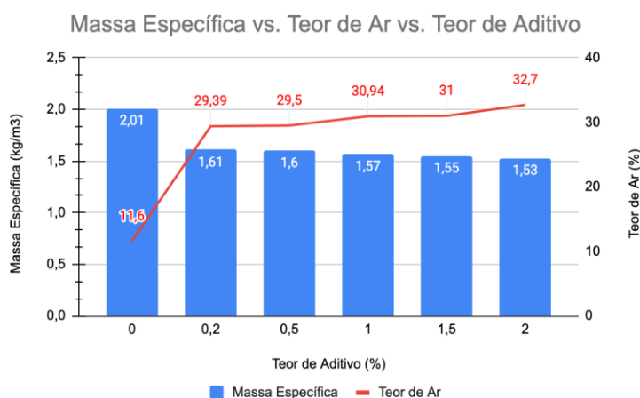
Gráfico 2 – Massa específica e teor de ar incorporado vs. concentração de aditivo
