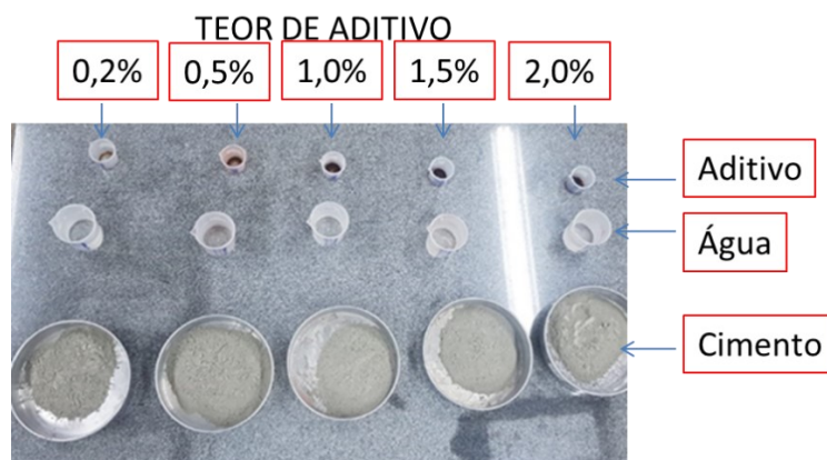
Figura 2 – Separação dos materiais para o preparo da argamassa
